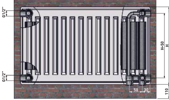
Termolux VK Ön Kesit Görünümü
