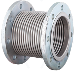
METAL KÖRÜKLÜ DÖNER FLANŞLI KOMPANSATÖRÜ
