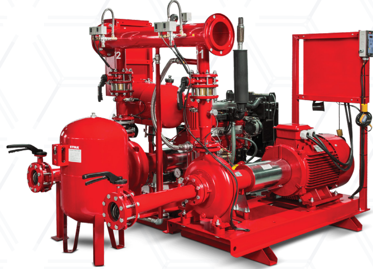
TS EN 12845 ST. YANGIN HİDROFORU
