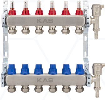
KARE TİP DEBİ VE TERMOSTAT AYARLI KOLLEKTÖR
