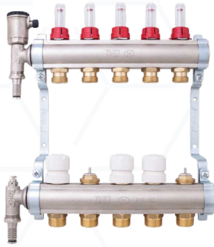
DEBİ VE TERMOSTAT AYARLI KOLLEKTÖR
