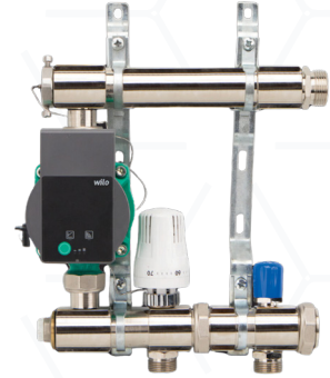
POMPALI KARIŞIM DEVRESİ
